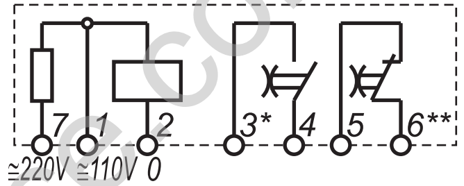
Рисунок 6 - Схема подключения реле ВЛ-65
