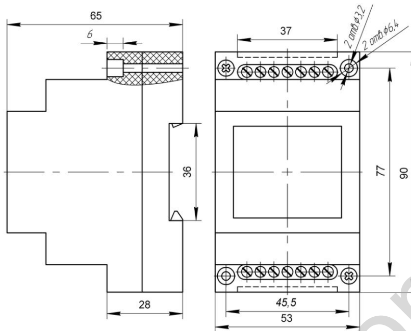
Рисунок 1 - Габаритные, установочные и присоединительные размеры реле
